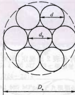
图 3 1×7 结构钢绞线外形示意图
