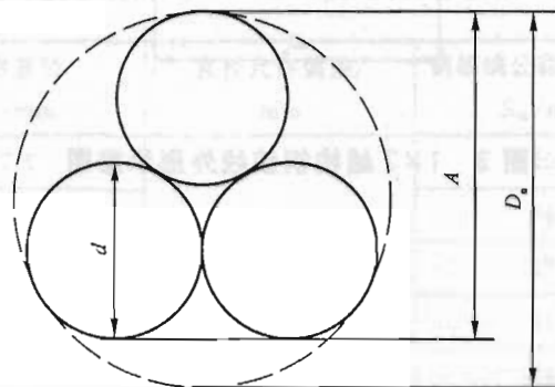
图 2 1×3 结构钢绞线外形示意图
