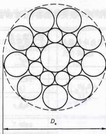
图 4 1×19 结构西鲁式钢绞线外形示意图
