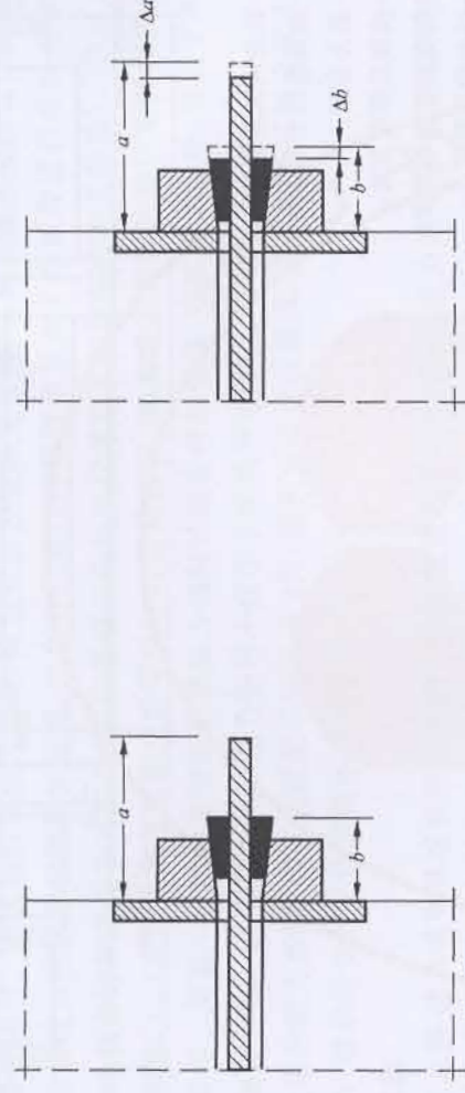
a) 锚固之前,预应力筋顶紧之后
