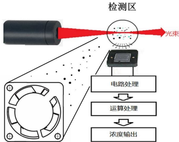
图 3-原理说明
