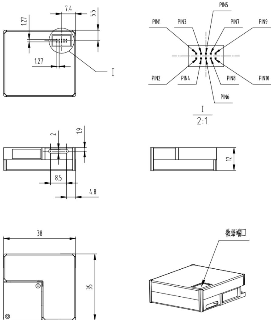
图 4-尺寸说明
