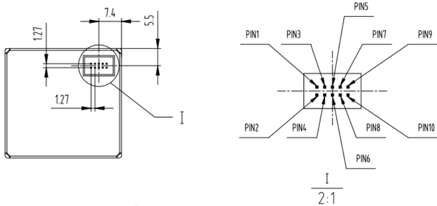
图 1-引脚顺序
