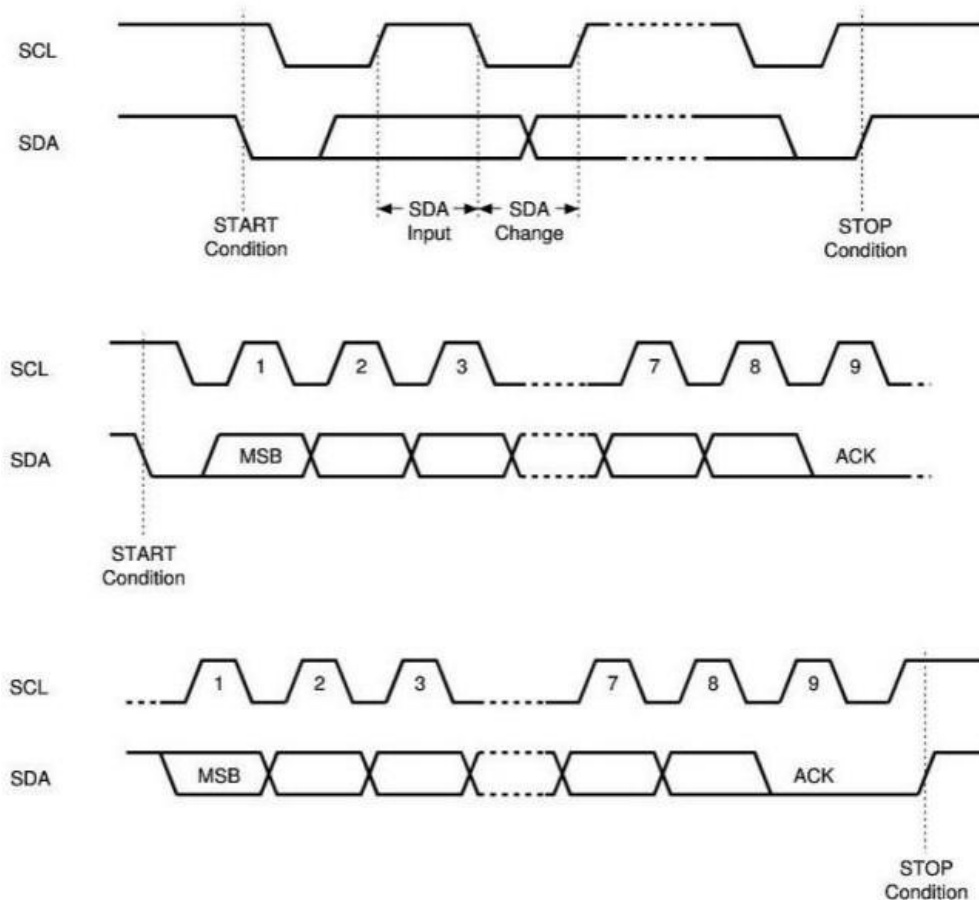
图 4 IIC 通讯协议
