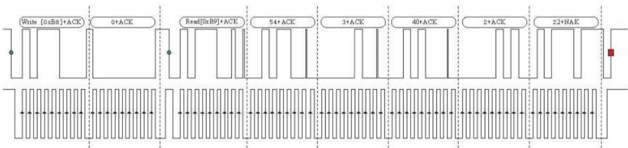
图 6: 参考时序图
