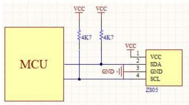
图 3: 应用电路
