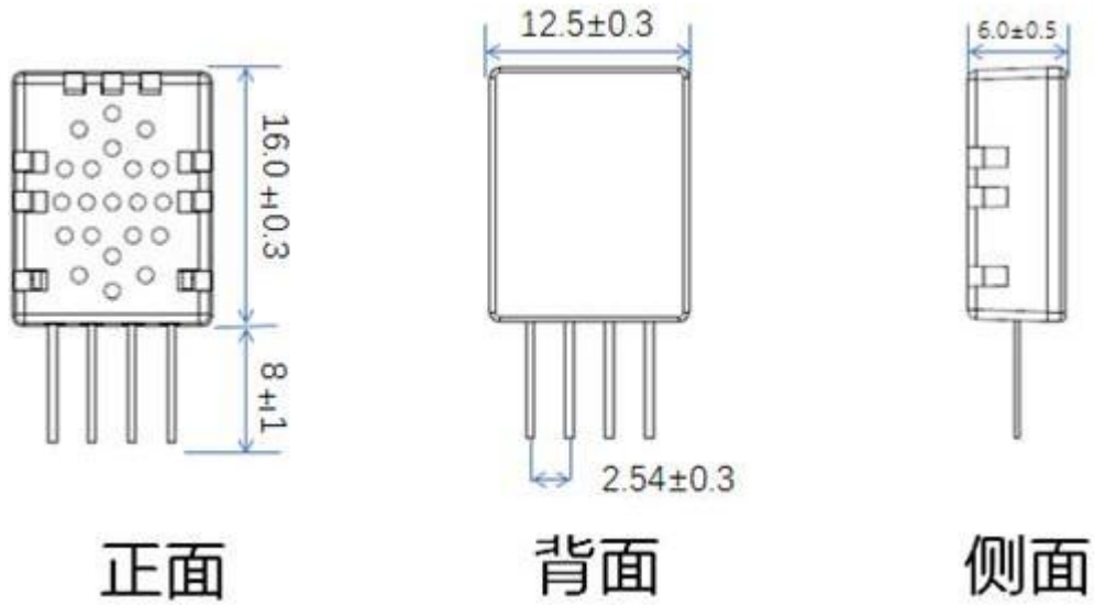
图 1: 温湿度模组结构图
