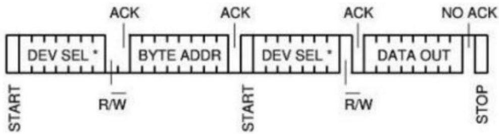
图 5: IIC 读取时序图
