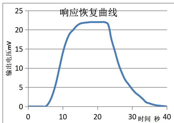
图4：响应恢复曲线
