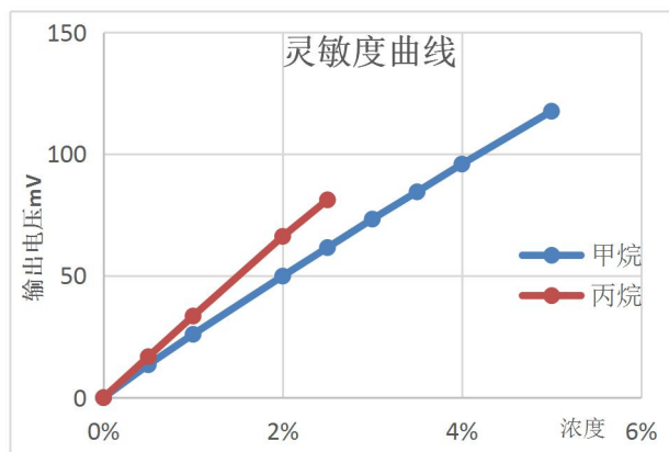
图3：灵敏度曲线
