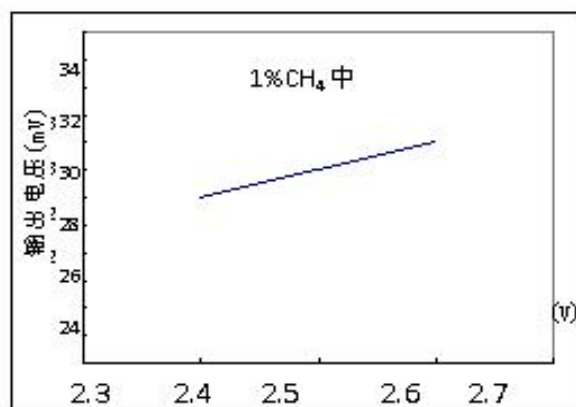
图 10：灵敏度电压波动特性曲线
