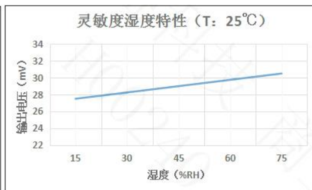
图8：灵敏度湿度特性曲线
