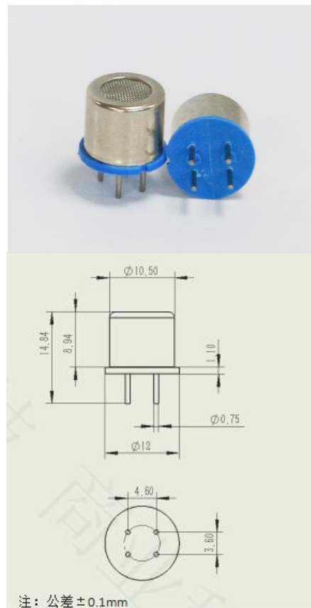
图 1：传感器外形结构
