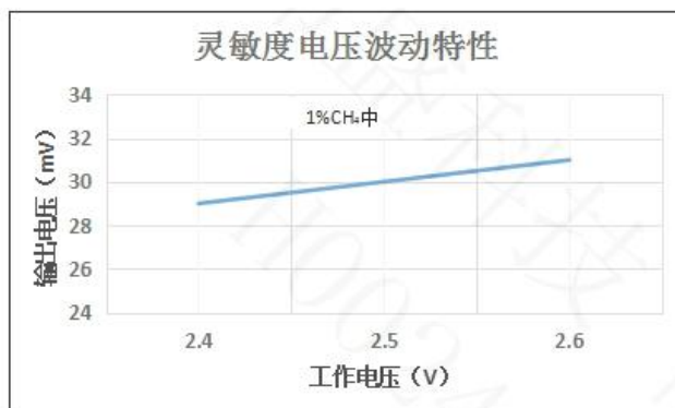
图 10：灵敏度电源波动特性曲线
