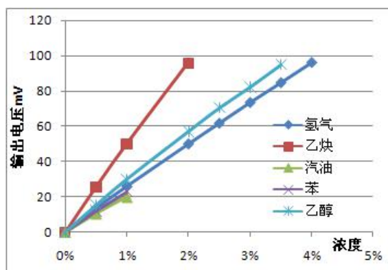
图 3: 灵敏度曲线
