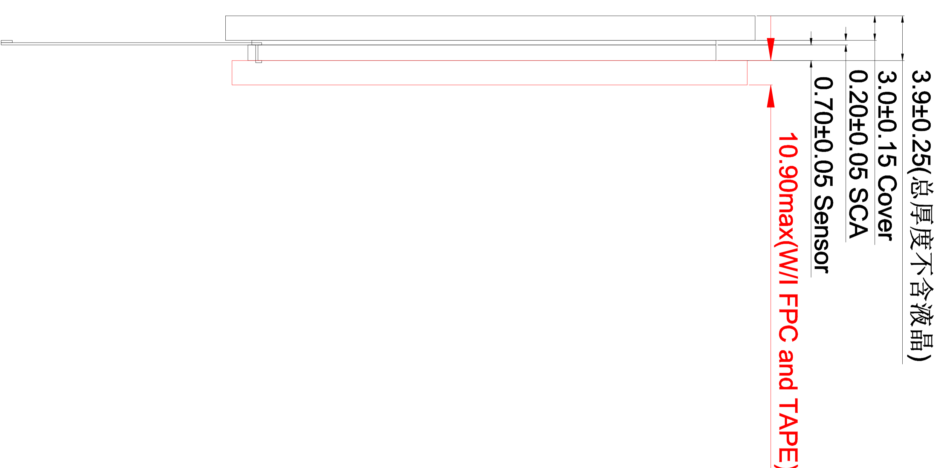
侧视图 横向10:1
