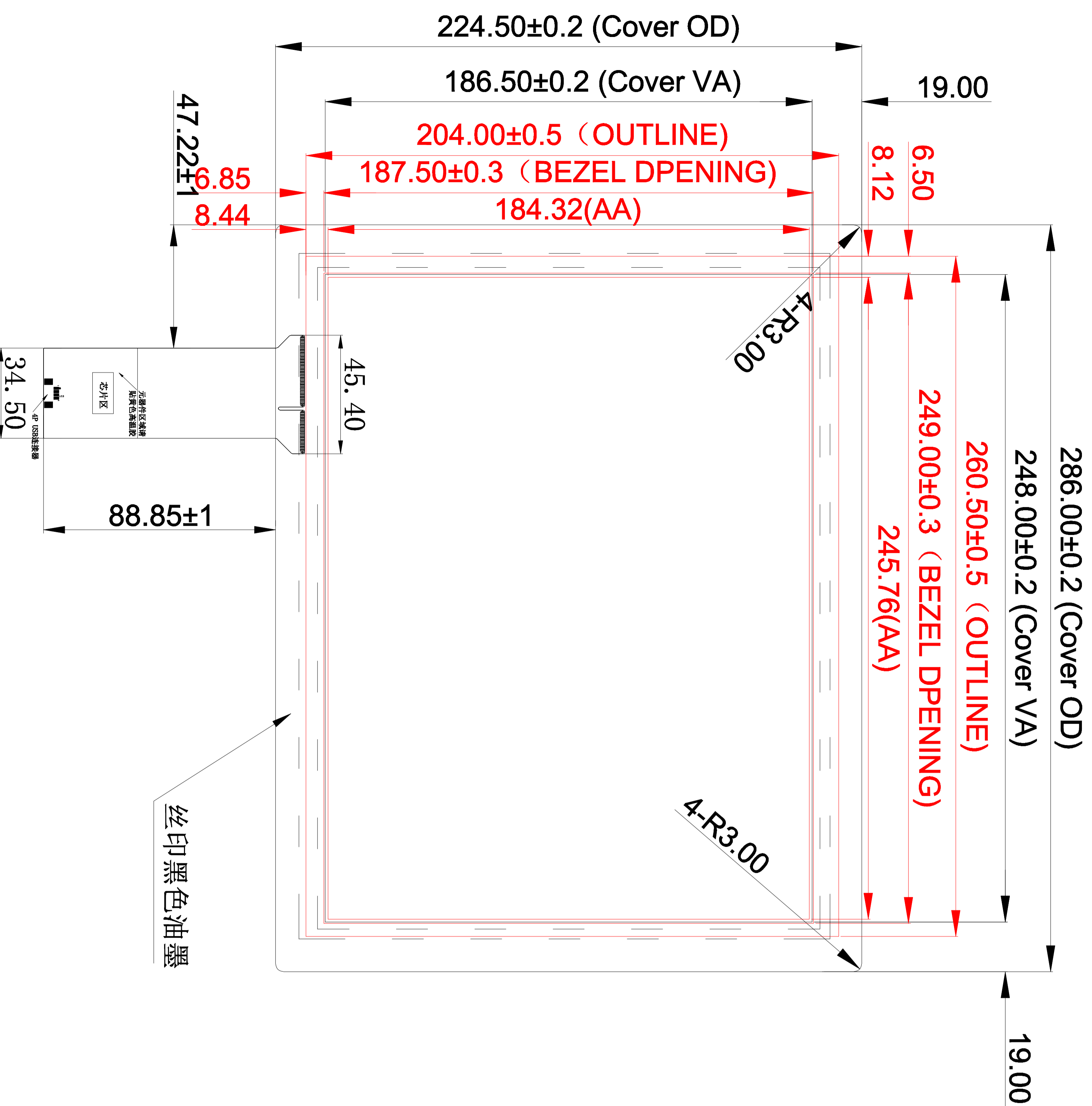
前视图 1:1
