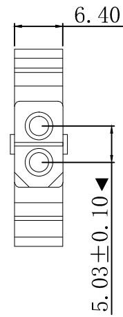
AH5031-02P AH5031NE-02P
