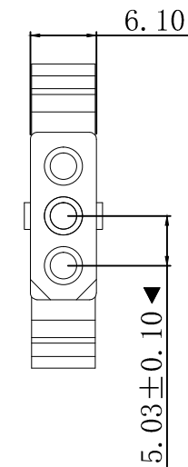
AH5031-03P AH5031NE-03P
