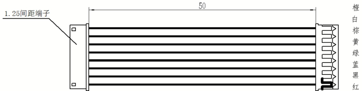
图3: Pin1.25mm*8 排线
